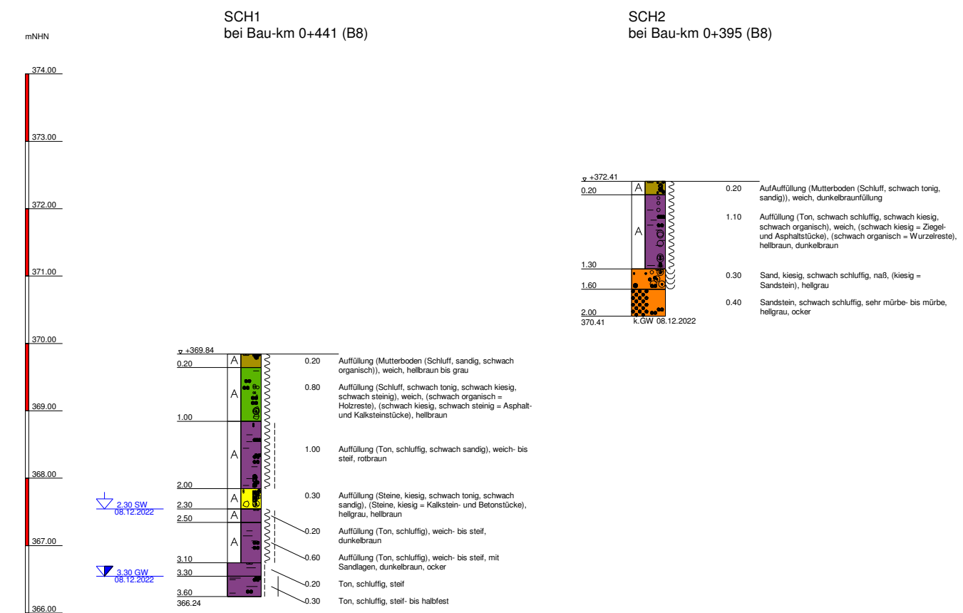
Schurprofil Maßstab 1:2,5
